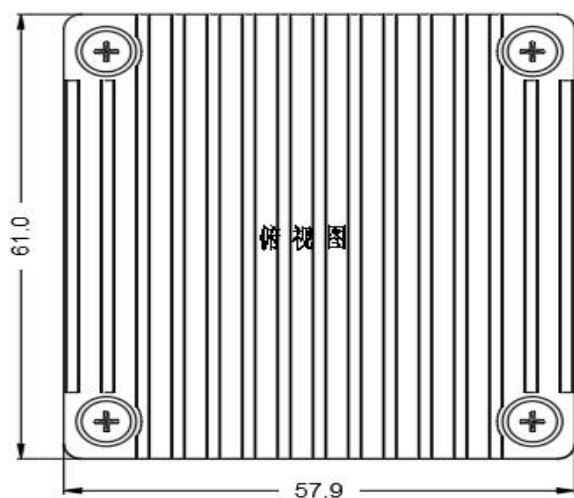
标准型+散热器 61.0*57.9*27.7mm
