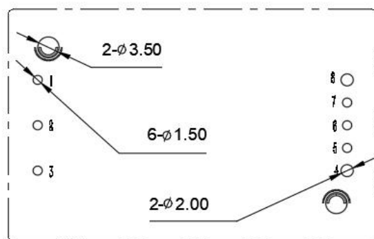
推荐PCB开槽尺寸
